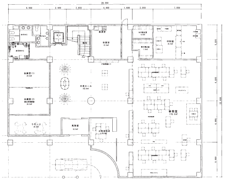
▲ 1階平面図
