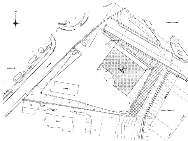
配置図（正面玄関は南西向き）
